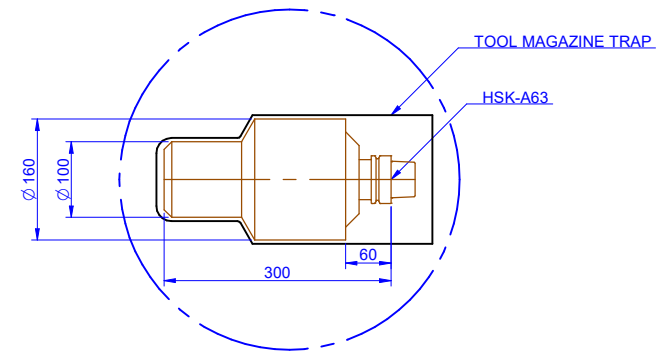
MAX. TOOL DIMENSIONS 1:5
