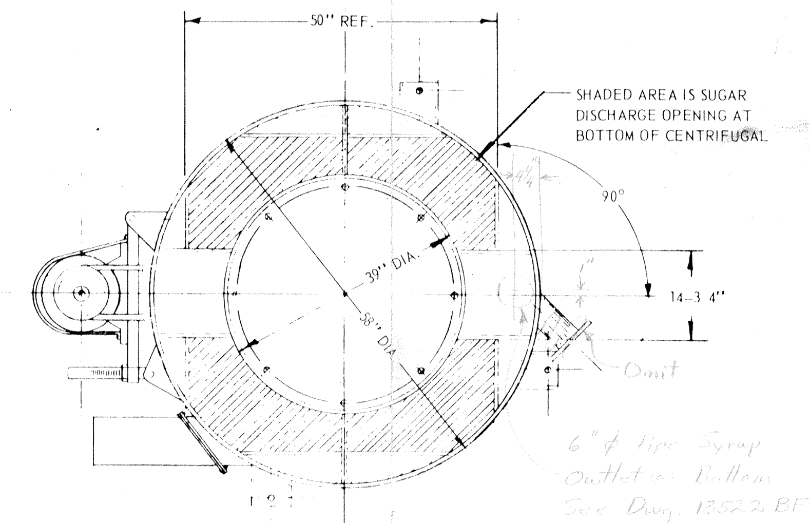
VIEW A-A
